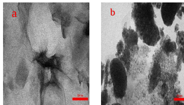
شکل ۳: تصاویر TEM از (a) \text{GO} و (b) هیبرید \text{H}_2 . خط مقیاس در (a) برابر با 300\text{ nm} و در (b) برابر با 100\text{ nm} می‌باشد.
