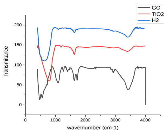
شکل ۴: طیف FTIR از \text{GO} ، \text{TiO}_2 و \text{H}_2 .
