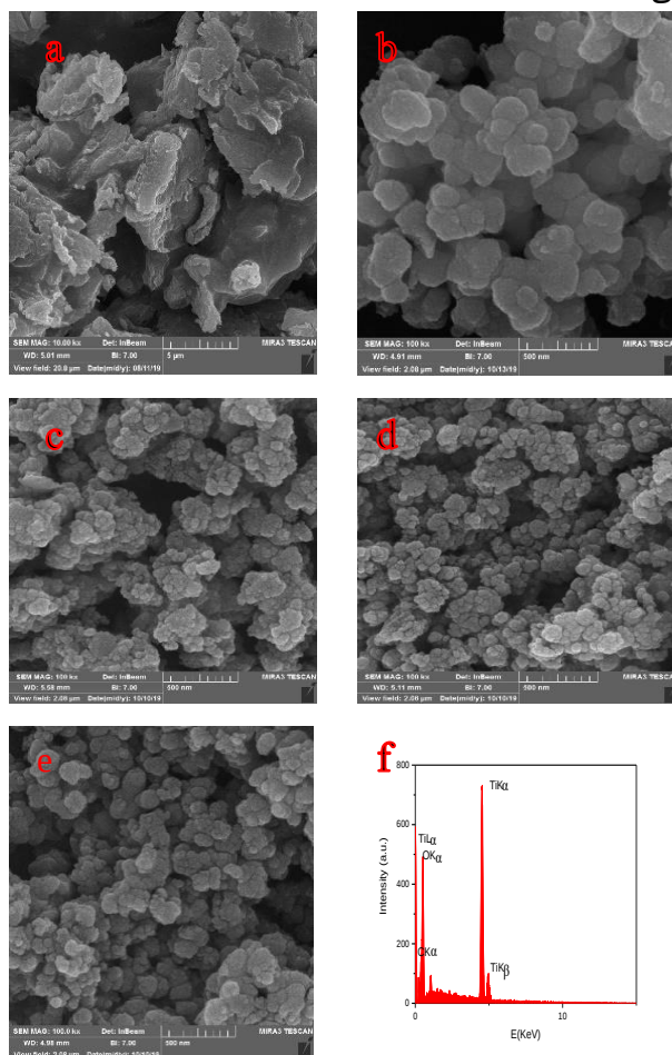
شکل ۲: تصاویر SEM از (a) \text{GO} ، (b) \text{TiO}_2 ، (c) \text{H}_1 ، (d) \text{H}_2 ، (e) \text{H}_3 و (f) نمودار EDX هیبرید \text{H}_2 .
