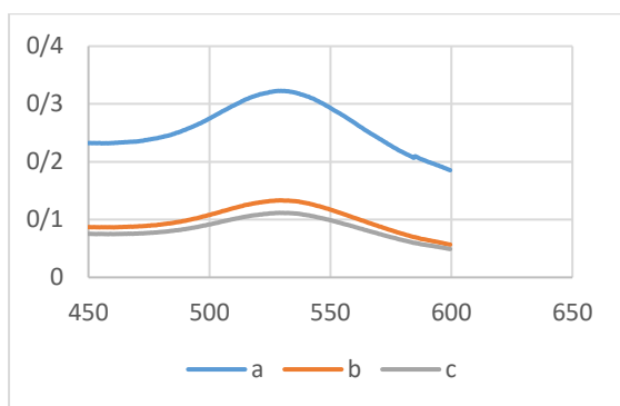
شکل (۴): نمودار جذب رزونانس پلاسمون‌های سطحی بر حسب طول موج برای گلوکز ۱۲۰. (a) نانوذرات طلا (b) نانوذرات طلا به همراه گلوکز (c) نانوذرات طلا به همراه گلوکز و گلوکز اکسیداز
