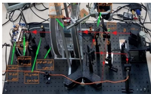
شکل ۵- تصویر چیدمان اپتیکی سیستم قفل طول موج به روش DAVLL
