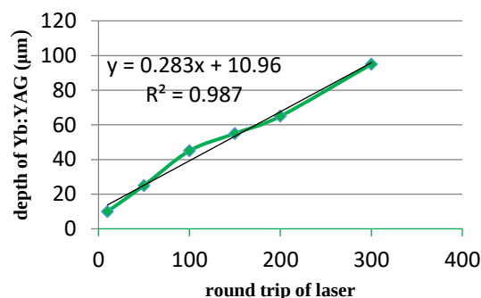
شکل ۳: نمودار تعداددرفت و برگشت پرتوی میکرولیزر بر روی کریستال برحسب عمق
