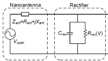
شکل (۱) مدار معادل سیستم رکت
