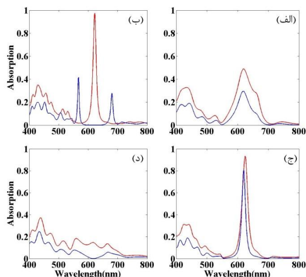
شکل ۲: طیف جذب (الف) و (ب) ساختار های ADPC به ترتیب با ضخامت نقص نیم موج و ربع موج (ج) و (د) ساختار های SDPC به ترتیب با ضخامت نقص نیم موج و ربع موج. در تمامی شکل ها رنگ قرمز و آبی به ترتیب برای نقص MDM و DMD می باشد.
