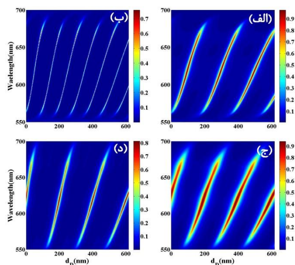
شکل ۴: تغییرات جذب با تغییر ضخامت نقص در ساختارهای
