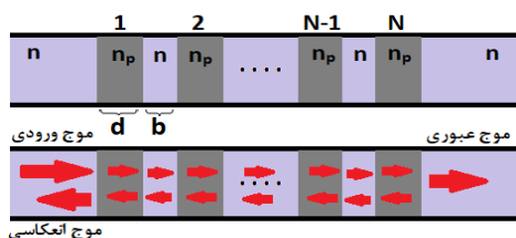
شکل ۱: (بالا) طرحواره ای از موجبر و N لایه قرار گرفته در آن. (پایین) موج فرودی به بلور فوتونی درون موجبر و بازتاب و عبور از لایه های آن.
