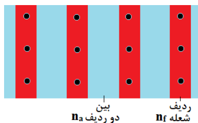
شکل ۳: شماتیکی از لایه‌های تناوبی ضریب شکست در فضای اشتعال (نقاط بیانگر موقعیت شعله‌ها می‌باشند).
