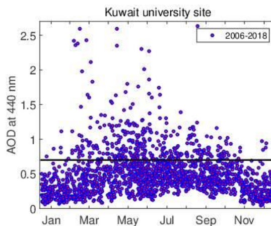
شکل ۲: عمق‌اپتیکی میانگین روزانه هواویزها در طول موج 440 nm از سال
