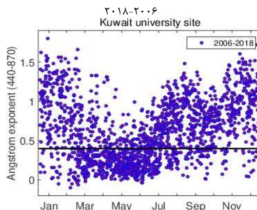
شکل ۳: نمای آنگستروم میانگین روزانه هواویزها از سال ۲۰۰۶-۲۰۱۸ برای ایستگاه شیدسنجی کویت. با توجه به شکل در ماه‌های مارس، آوریل، می، ژوئن و جولای ذرات درشت غبار به جو اضافه می‌شوند.
