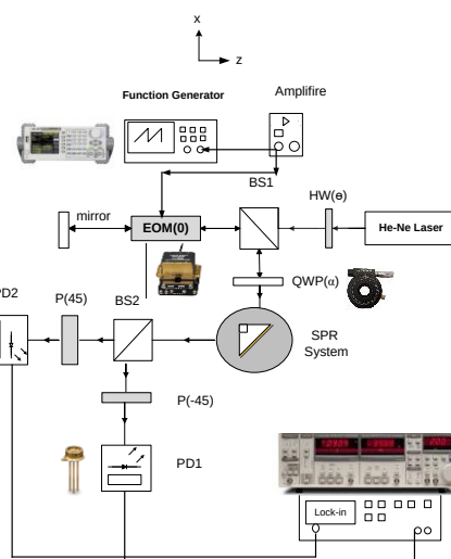
شکل ۲: طرح شماتیک چیدمان تداخل سنجی قطبشی هتروداين مسیر مشترک
