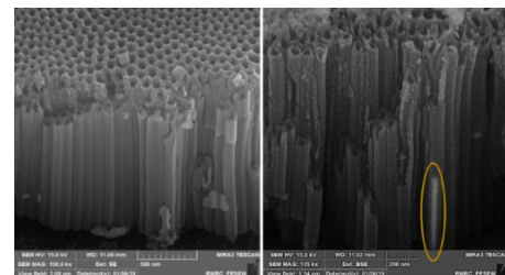
شکل ۱: تصویر FESEM از سطح مقطع نمونه سنتز شده، (الف) چیدمان منظم نانولوله‌ها به خوبی مشخص است. (ب) نانومیل نقره در درون نانولوله تشکیل شده است [۶].
