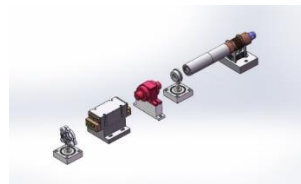
شکل ۲: طرحواره‌ی از سیستم دوبار عبور تقویت کننده فلش لامپ میکرولیزر سوئیچ Q انفعالی.
