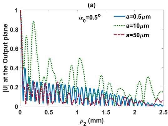
شکل ۲: پروفایل عرضی مد غالب رزوناتور را نشان می‌دهد که بر حسب پارامتر هایپربولیید خیلی کوچک رسم شده است.
