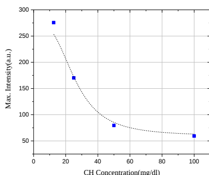
شکل ۳: محنی شدت بیشینه طیف فوتولومینسانس کلسترول بر حسب غلظت.
