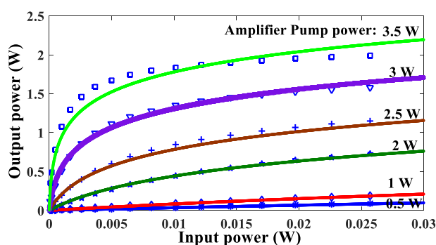
شکل ۳: نمودار توان‌های ورودی به توان خروجی برحسب توان‌های مختلف دهمش تقویت کننده
