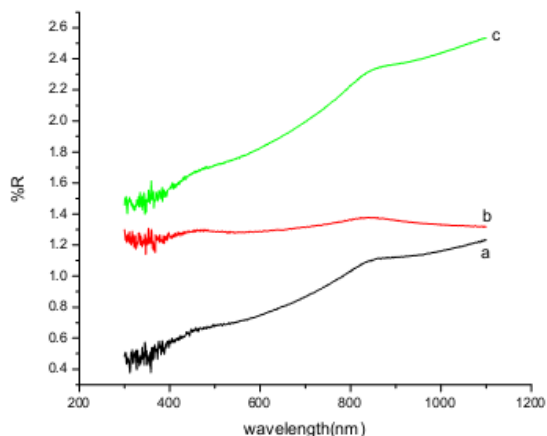
شکل ۳. طیف بازتابی نانوذرات آلاییده با نسبت های مختلف بورن: (a) ۱٪، (b) ۳٪، (c) ۵٪
