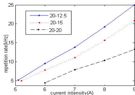
شکل ۶: تغییرات نرخ تکرار بر حسب شدت جریان لیزر دیود به ازای پهنای تپ جریان ثابت 60 \mu\text{s} برای هر سه سامانه اپتیکی در دمای 45.5^\circ\text{C} لیزر دیود
