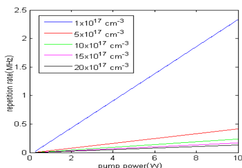
شکل ۳: تغییرات نرخ تکرار بر حسب توان دمش به ازای غلظت های مختلف آرایش جاذب اشباع پذیر
