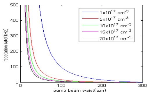
شکل ۲: تغییرات انرژی تپ، پهنای تپ و نرخ تکرار بر حسب شعاع پرتو دمش به ازای غلظت های مختلف آرایش جاذب اشباع پذیر
