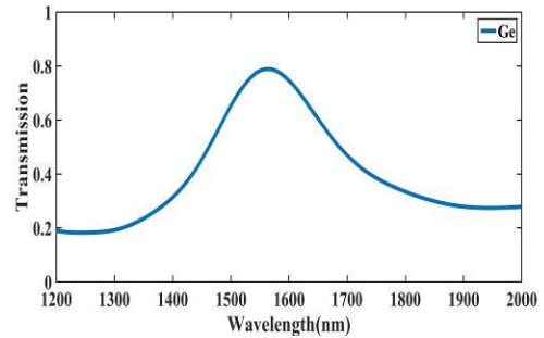
شکل ۲. نمودار طیف عبور هنگامیکه از آرایه متناوب با ثابت شبکه ۴۴ نانومتر از نانوذراتی کروی از جنس نقره با شعاع ۱۱ نانومتر داخل لایه‌ی از ژرمانیوم با ضخامت ۳۵۵ نانومتر قرار داده ایم.
