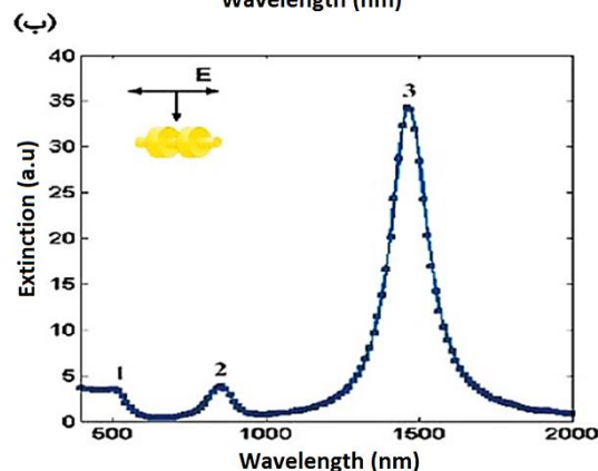
شکل ۶: الف) نتایج شبیه‌سازی طیف سطح مقطع خاموشی نانوساختار پیشنهادی (آبی) و نانوکره با شعاع ۵۰ nm (سبز)، در هوا (RI=۱) با L_2=50 nm، L_1=40 nm و \Delta R=60 nm، و d_1=40 nm. قله‌های تشدید در طول موج‌های \lambda_1=507 nm و \lambda_2=856 nm ب) و سومین قله‌ی تشدید LSPR غالب در \lambda_3=1460 nm رخ می‌دهد.
