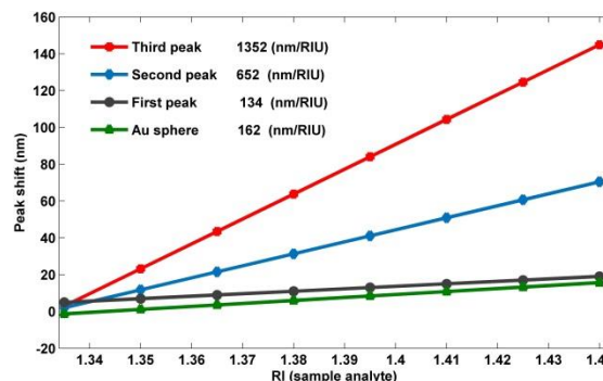
شکل ۵: نمودار جایجایی قله‌های تشدید LSPR بر حسب تغییر ضریب شکست محلول زیستی پیرامون نانوساختار. طبق شکل به ترتیب برای قله‌ی اول تا سوم در طیف سطح مقطع خاموشی نانوساختار پیشنهادی حساسیت‌های ۱۳۴ nm/RIU (خاکستری)، ۶۵۲ nm/RIU (آبی)، ۱۳۵۲ nm/RIU (قرمز) و برای نانوکره طلا با شعاع ۵۰ nm حساسیت ۱۶۲ nm/RIU (سبز) به دست آمده است.
