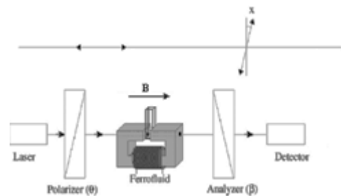
شکل ۱: چیدمان فارادی.
