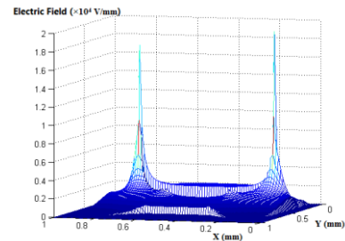
شکل ۷: شکل سه‌بعدی تغییرات میدان الکتریکی در مدل پیش یونش ردیف جرقه. محور عمودی مربوط به میدان الکتریکی ( 10^4 \text{ V/mm} ) است.
