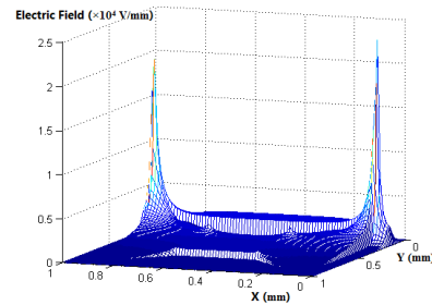
شکل ۶: شکل سه‌بعدی تغییرات میدان الکتریکی در مدل پیش یونش کرونا. محور عمودی مربوط به میدان الکتریکی ( 10^4 \text{ V/mm} ) است.
