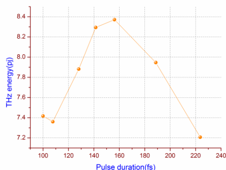
شکل ۲: شدت تابش تراهرتز برای پالس‌های با انرژی ۴ میلی‌ژول، بدون چیرپ و پهنای زمانی ۱۰۰، 107/7 ، 128/06 ، 141/42 ، 156/2 و 188/68 فمتوثانیه
