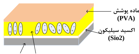
شکل ۳: شکل لایه‌های فیلم نازک پلیمر برای ساخت موجبر ماخزرنر.
