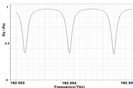
شکل ۸ پاسخ فرکانسی تشدیدگر با شعاع ۳cm- ضریب تزویج ۰,۰۵db/cm- تلفات ۰,۰۵db/cm
