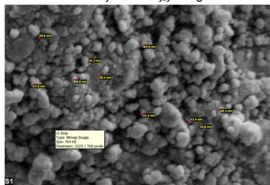
شکل ۳: تصویر (SEM) نمونه LZCF
