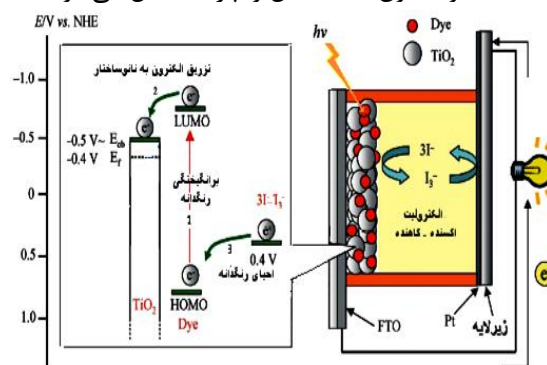
شکل ۱: ساختار DSSC و چرخه الکترون در آن ۱. برانگیختگی رنگدانه، ۲. تزریق الکترون به \text{TiO}_2 ، ۳. احیای رنگدانه.
