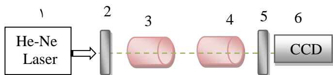
شکل ۲: چیدمان قطبش نگاری، لیزر هلیوم نئون موازی شده، ۲ و ۵ قطبیده و واکافنده، ۳ و ۴ میله لیزر Nd:YAG، ۶: CCD
