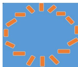
شکل ۷: جهت‌گیری دایرکتورها درون یک لایه کریستال مایع (از نمای کنار).
