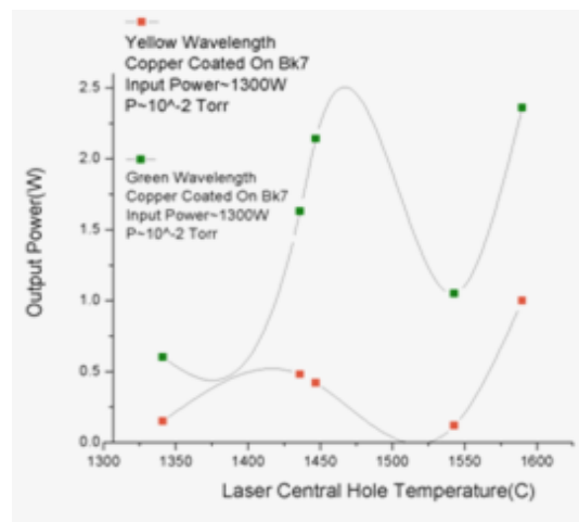
شکل ۵: توان خروجی طول موج زرد لیزر بخار مس در حفره مرکزی با آینه مسی و زیر لایه BK7 در فشار 10^{-2} Torr. سبز: توان خروجی طول موج سبز لیزر بخار مس با آینه مسی در حفره مرکزی در فشار 10^{-2} Torr.
