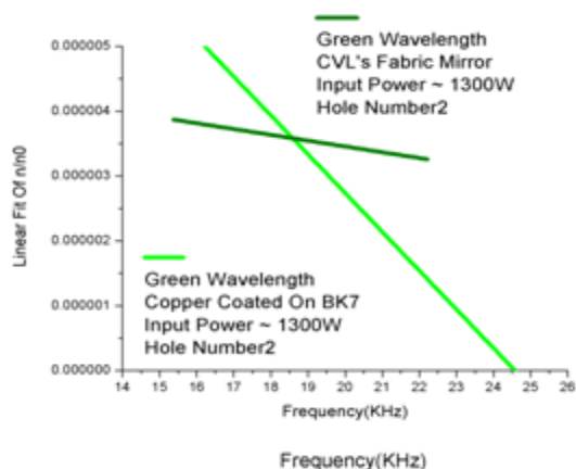
شکل ۶: نمودار فرکانس بر حسب n/n_0 برای طول موج سبز روزنه دوم در فشار 10^{-2} Torr و توان ورودی حدود 1300W .
