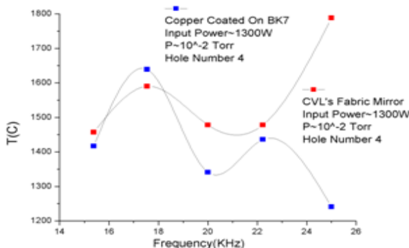
شکل ۴: دمای دیواره لیزر بخار مس با آینه اصلی لیزر در فشار 10^{-2} Torr و با فرکانس‌های مختلف. آبی: دمای لیزر بخار مس با آینه مسی و زیر لایه BK7 در فشار 10^{-2} Torr در همان فرکانس‌ها.
