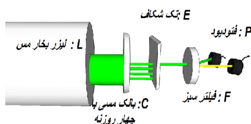
شکل ۲: چیدمان آزمایشگاهی برای اندازه‌گیری دمای پلاسما مس داخل تیوب لیزر
