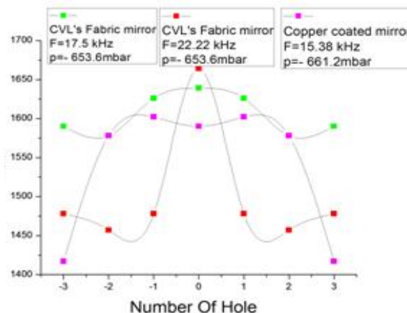
شکل ۳: نمایه دمایی لیزر بخار مس با آینه اصلی لیزر در فرکانس 22.2 kHz در فشار 10^{-2} Torr؛ سبز: فرکانس 17.5 kHz در فشار 10^{-2} Torr؛ بنفش: نمایه دمایی لیزر با آینه مسی در فرکانس 15.38 kHz در فشار 10^{-2} Torr.
