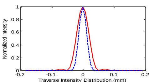
شکل ۴: توزیع شدت عرضی در صفحه کانون (میلی‌متر). نمودار خط‌چین مربوط به پهنای ۸و۶،۴ و نمودار با خط صاف مربوط به پهنای ۱۰و۶،۴ MFZP است. پهنای این پرتوگوسی به ترتیب ۱۰۰ و ۱۰۰ میکرومتر است.
