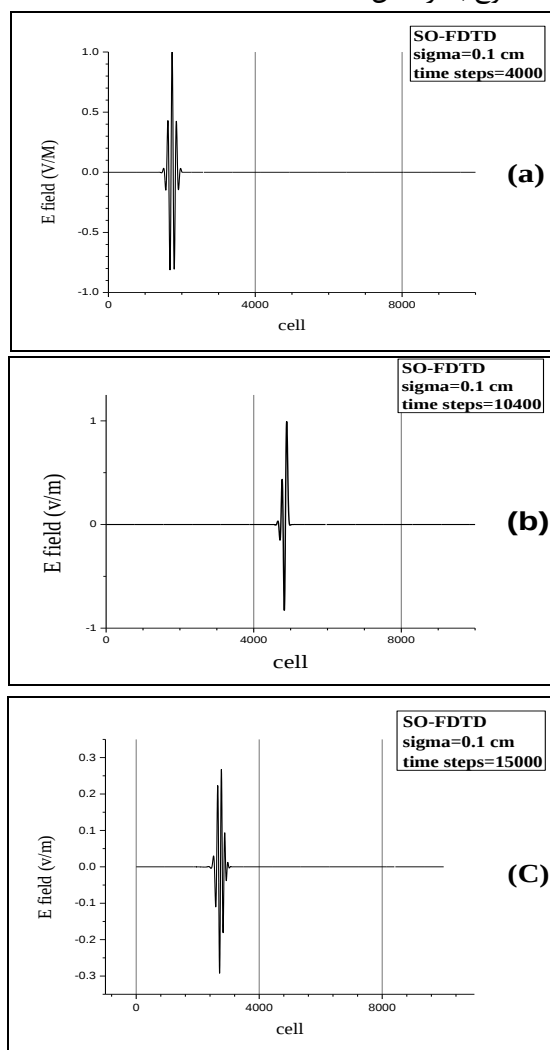
شکل ۲: انتشار موج با فرکانس 0.1 THz و پلاسما با \sigma = 0.1 \text{ cm} . (a) گام زمانی ۴۰۰۰، (b) گام زمانی ۱۰۴۰۰، (c) گام زمانی ۱۵۰۰۰.
