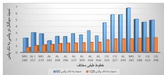
شکل ۵: نمودار نسبت شدت تابش پلاسما در حالت دو پالسی (۳۰+۹۰ میلی ژول، \Delta T=100 ns) به حالت تک پالس (۱۲۰ و ۶۰ میلی ژول)
