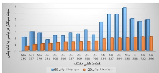
شکل ۵: نمودار نسبت شدت تابش پلاسما در حالت دو پالسی (۳۰+۹۰ میلی ژول، \Delta T=100 ns) به حالت تک پالسی (۶۰ و ۱۲۰ میلی ژول)
