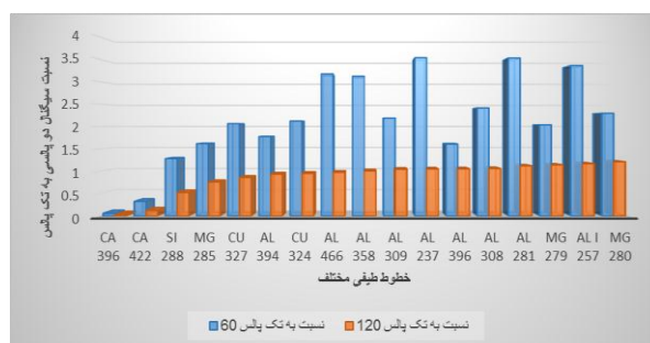
شکل ۴: نمودار نسبت شدت تابش پلاسما در حالت دو پالسی (۳۰+۹۰ میلی ژول، \Delta T=100 ns) به حالت تک پالس (۶۰ و ۱۲۰ میلی ژول)
