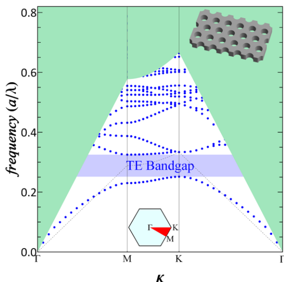
شکل ۱: ساختاربانند TE-like شبکه پایه ای که ابر بلور خود را روی آن می سازیم. تیغه بلور پایه در گوشه بالا سمت راست شکل دیده می شود. خط چین سیاه مخروط نور ابر بلور است.
