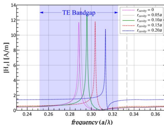
شکل ۲: اندازه مولفه z میدان مغناطیسی در نقطه ای نزدیک به کاواک و در صفحه میانی تیغه بر حسب فرکانس برای کاواک ها با شعاع مختلف. ناحیه آبی رنگ بیانگر گاف بلور پایه است
