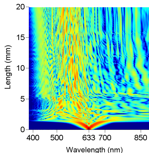
شکل ۵: طیف ابرپیوستار در محدوده نور مرئی در طول ۲۰ میلی‌متر از فیبر بلور فوتونی.
