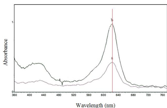
شکل ۱: طیف جذبی برای (a) مالاچیت گرین، (b) زوج یون اورانیوم بنزوات با مالاچیت گرین در کلروفرم و اتانول. خط جذب اورانیوم در ۶۲۲ قرار دارد.
