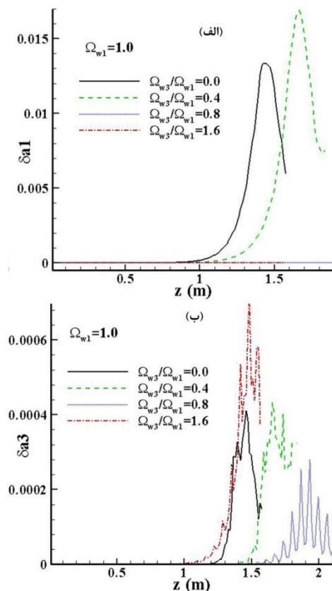
شکل ۱. تغییرات تابش (الف) فرکانس اصلی و (ب) هارمونیک سوم بر حسب z در ویگلر تعمیم‌یافته برای مقادیر مختلف میدان هارمونیک
