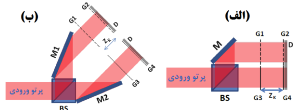
شکل ۳: دو آرایش به کار رفته در مطالعه اثر انعکاس: M آینه، توری، BS پرتوشکن، D صفحه مات.
