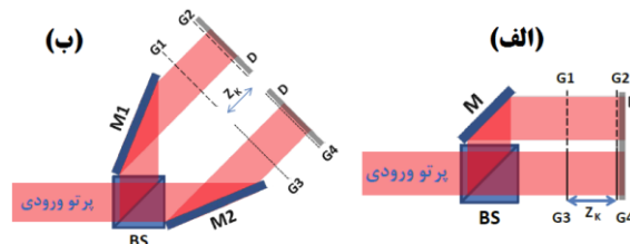
شکل ۳: دو آرایش به کار رفته در مطالعه اثر انعکاس: M آینه، توری، BS پرتوشکن، D صفحه مات.
