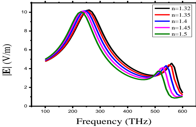
شکل ۳-الف. نمودار تشدید نانوانتِن پاپیونی با قطبش نور فرودی در جهت x با مقادیر مختلف ضرایب شکست برای محیط اطراف
