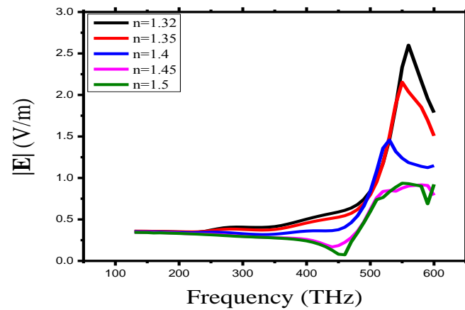
شکل ۳-ب. نمودار تشدید نانوانتِن پاپیونی با قطبش نور فرودی در جهت z با مقادیر مختلف ضرایب شکست برای محیط اطراف
