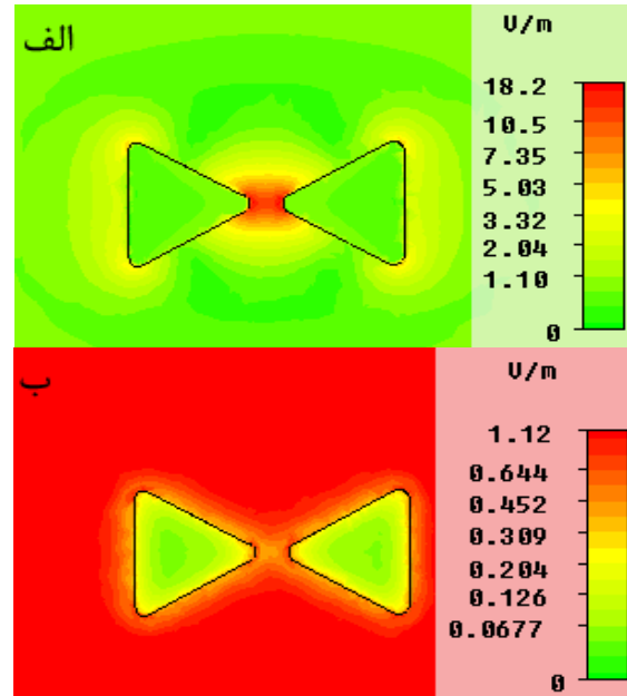
شکل ۲- توزیع میدان الکتریکی در اطراف نانوانتِن پاپیونی. (الف) قطبش نور فرودی موازی با طول بلند نانوانتِن (ب) قطبش نور فرودی عمود بر طول بلند نانوانتِن
