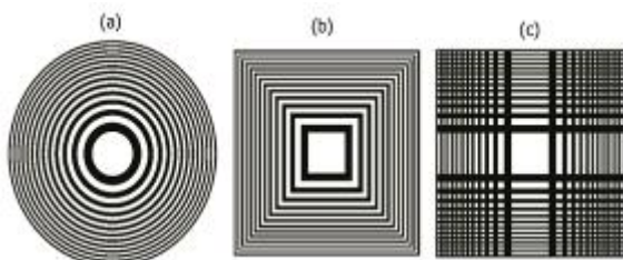
شکل (۱): ساختار تیغه‌ی منطقه‌ای فرنل (a) دایره‌ای، (b) مربعی و (c) صلیبی شکل
