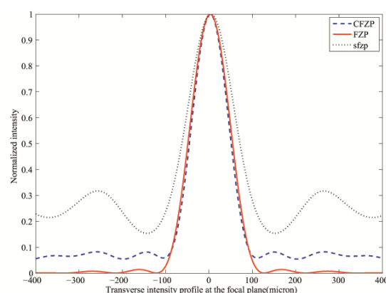
شکل (۳): توزیع شدت بهنجار شده‌ی سه عنصر پراشی مذکور در صفحه‌ی کانون
