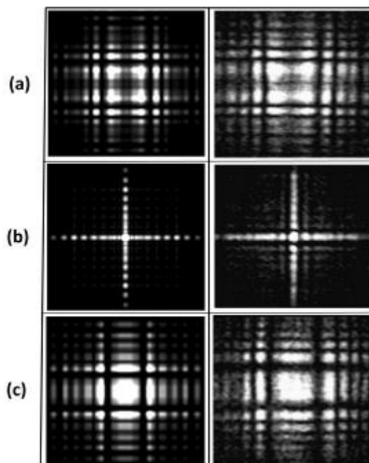
شکل (۷): دامنه‌ی میدان پراشی عنصر صلیبی شکل در صفحه‌ی کانونی که اولین ستون از سمت راست به صورت تجربی و دومین ستون به صورت شبیه‌سازی ثبت شده است. به ترتیب سطر ۱ تا ۳، ۲۰۰، ۲۰۰ میلیمتر قبل از کانون، در کانون و ۲۰۰ میلیمتر بعد از کانون می‌باشند.
