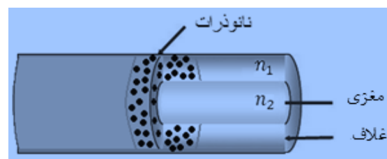
شکل ۱: شماتیک کلی فیبر با غلاف کامپوزیت
