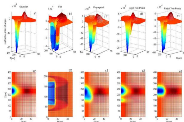
شکل ۳: پروفایل فضایی مولفه X تغییرات ضریب شکست (a-e)، بعد از گذر پالس برای توزیع های دمایی متفاوت در ناحیه کانون 4.5ns
