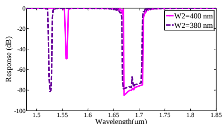
شکل ۳: پاسخ درگاه انتقال فیلتر افزایشی-کاهشی با توری براگ ایجاد شده بر روی دیواره موجبرهای نواری به ازای مقادیر متفاوت از W_2 .
