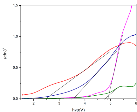
شکل ۴: منحنی (\alpha hv)^2 بر حسب h\nu
