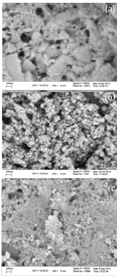
شکل ۶: (a) نمونه بدون اولئیک اسید. (b) نمونه تهیه شده با افزودن ۱۰/۶ ml اولئیک اسید. (c) نمونه تهیه شده با افزودن ۱۰/۰ ml اولئیک اسید
