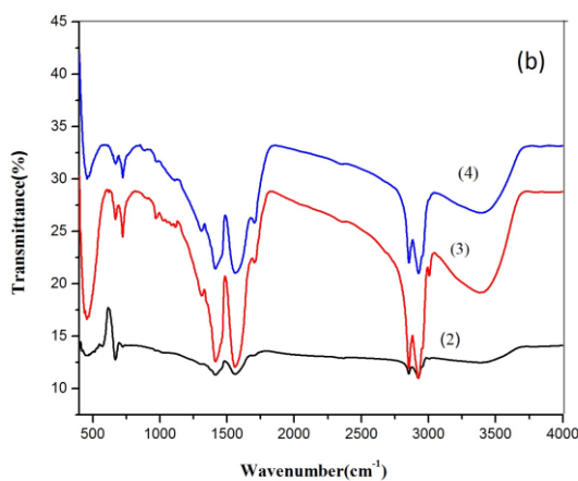
شکل ۵: (a) طیف FTIR مربوط به نمونه بدون اولئیک اسید. (b) طیف FTIR مربوط به نمونه‌های تهیه شده با غلظت‌های مختلف اولئیک اسید (۱) ۰ ml (۲) ۰/۲ ml (۳) ۰/۶ ml (۴) ۱ ml
