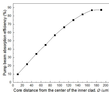
شکل ۳: تغییرات جذب پرتو دمش نسبت به \rho در تار دوغلافی با سطح مقطع دایره‌ای با شعاع غلاف داخلی R = 200 \mu\text{m} و شعاع هسته r_0 = 6 \mu\text{m}
