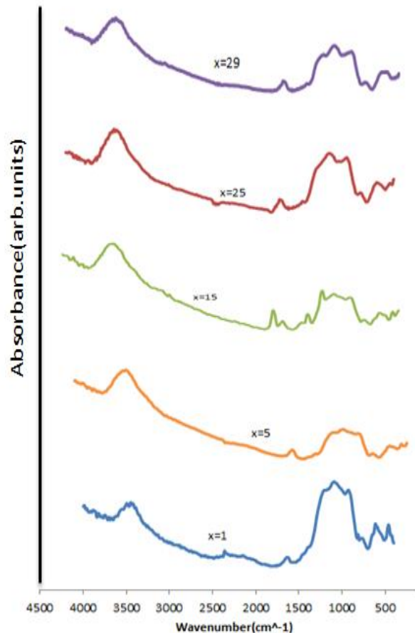
شکل ۶: طیف فرسرخ نمونه ها
