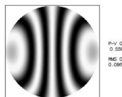
شکل ۹: الگوی تداخلی بیانگر افت کیفیت در سامانه، در نتیجه‌ی ایجاد عدم هم‌راستایی به میزان TLB=0,1^\circ در لنز اول
