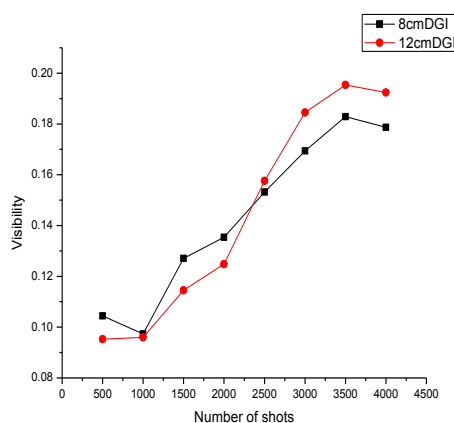
شکل ۵: نمودار تباین نسبت به شات برای طول های محفظه با x=8,12\text{cm}
