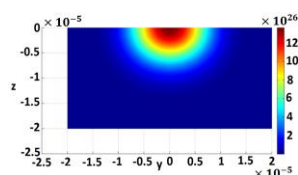
شکل ۲: توزیع عرضی غلظت تیتانیوم در موجبر کانالی با شرایط نفوذ W = 10 \mu\text{m} ، t = 180 \text{ nm} ، t = 17 \text{ h} ، T = 1050^\circ\text{C} .
