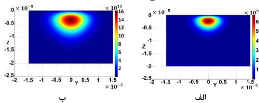
شکل ۴: توزیع میدان الکتریکی مد TM_{00} (الف) و TE_{00} (ب) در موجبر کانالی با همان شرایط نفوذ.
