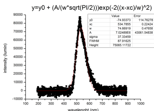
شکل ۷: طیف الکترو لومینسانس قطعه ب متصل شده به ولتاژ ۱۲ ولت
