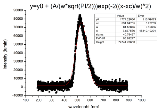
شکل ۶: طیف الکترو لومینسانس برای قطعه الف متصل به ولتاژ ۷ ولت
