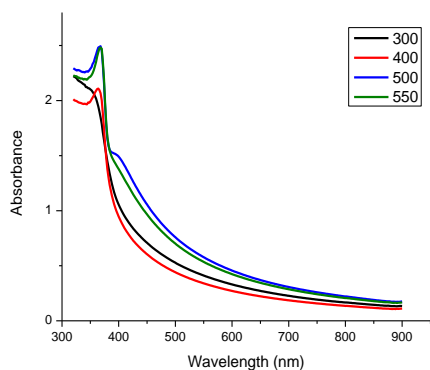
شکل ۴ طیف جذبی نمونه های ZnO بازیخت شده در دماهای مختلف
